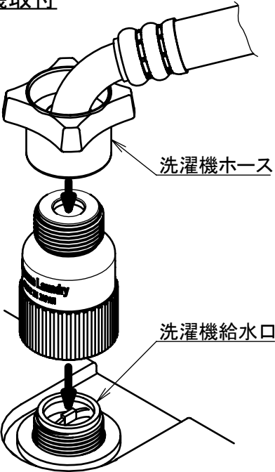
洗濯機取付
